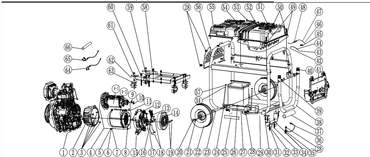
10001-03841-00爆炸图 SCD11000E
