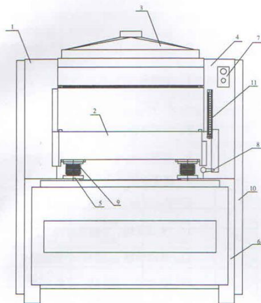
一、机床外形结构图(1)
