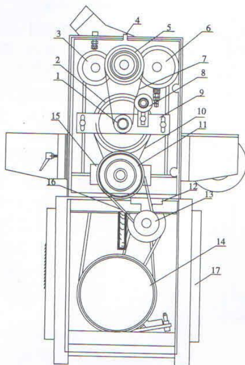
机床外形结构图 (3)
