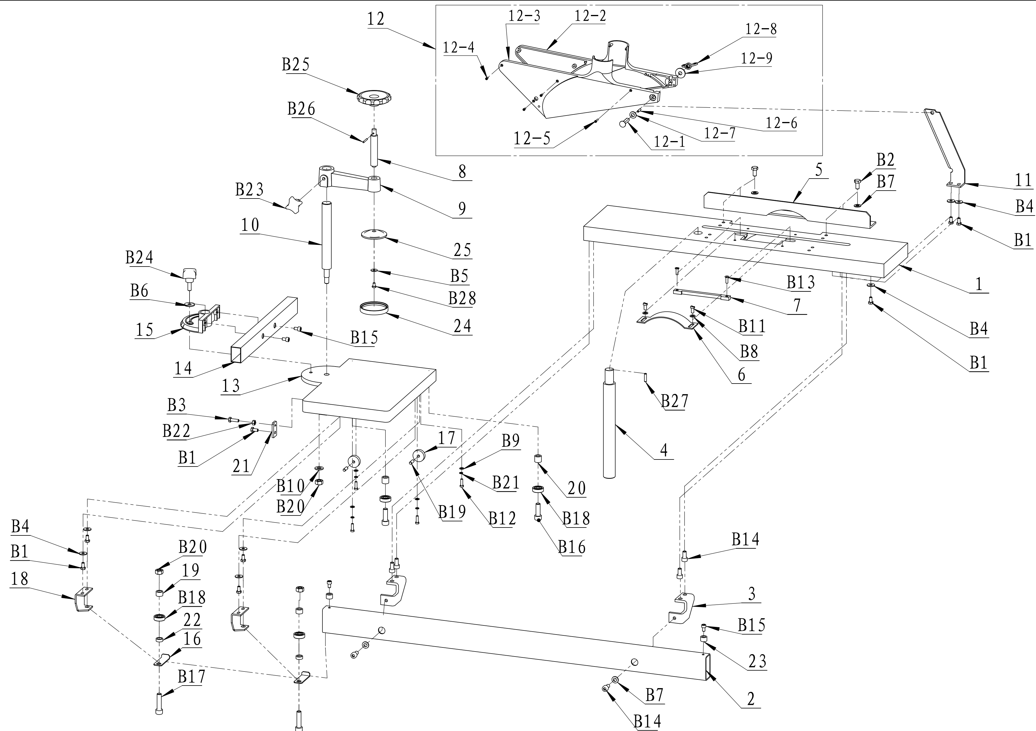
圓鋸工作台部分 ML393A. LT04
