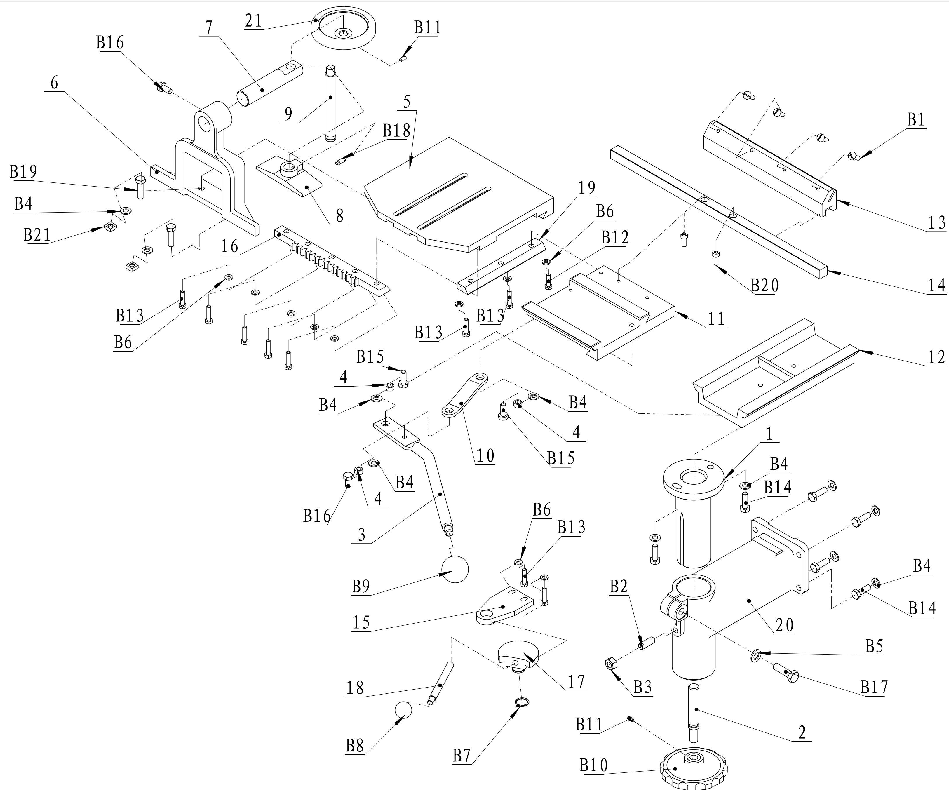
榫槽部分 ML393A. LT06
